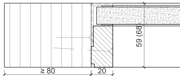
Glasleiste einseitig bündig Metallwinkel
