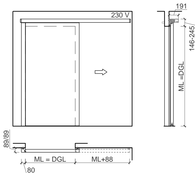
Anschlag(Horizontalschnitt)
