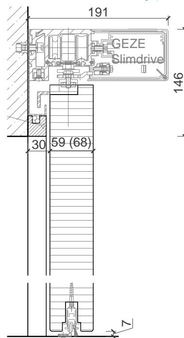
Antrieb und Bodenführung (Vertikalschnitt)
